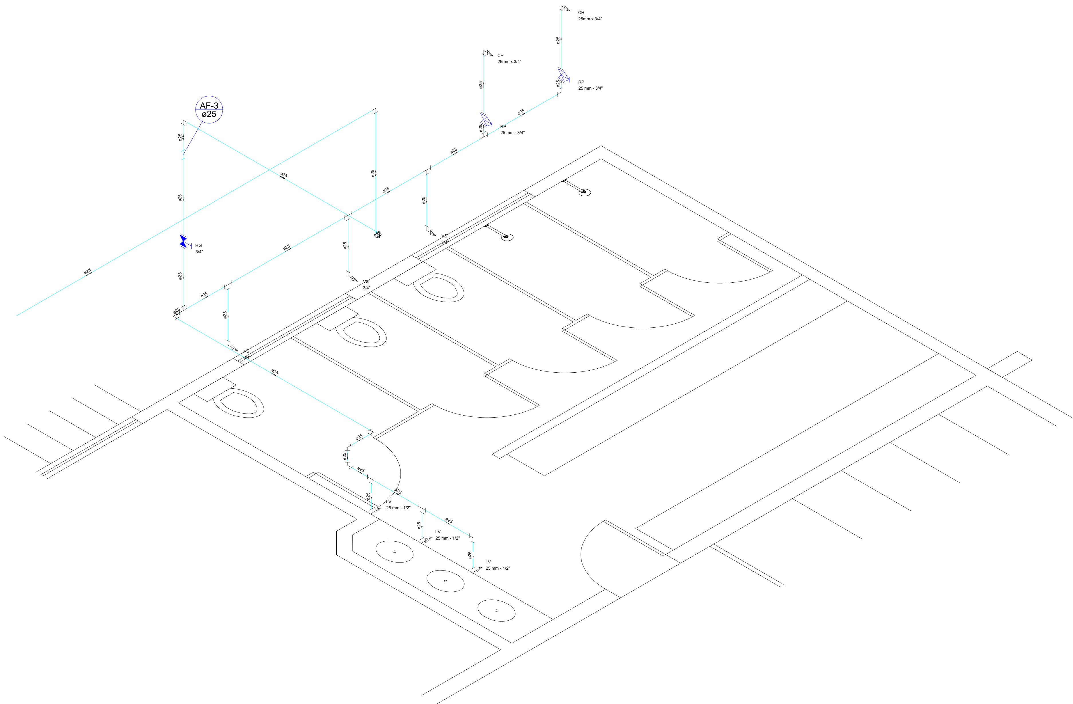
Detalhe H3 escala 1:25
